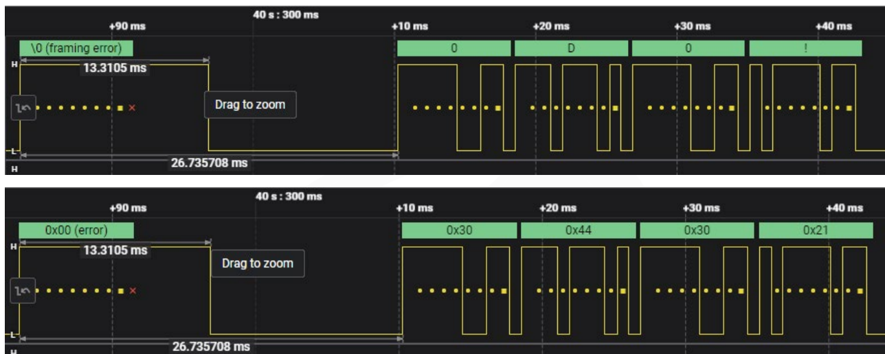
图13. 波形图
